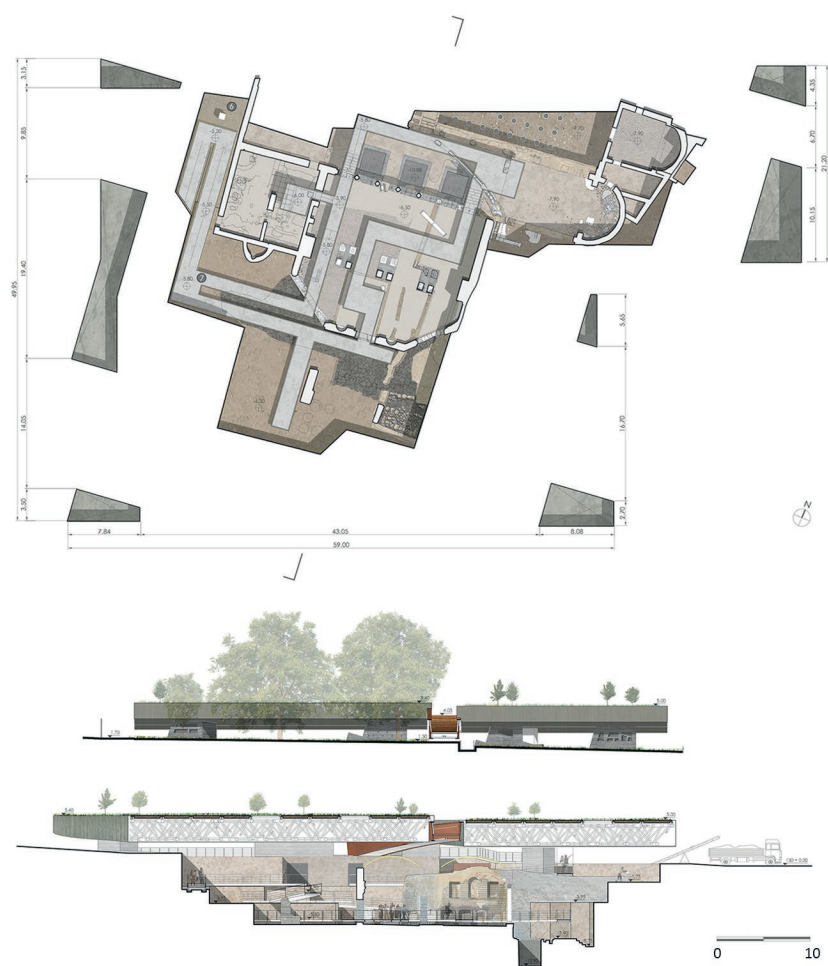
Fig. 4 - (A partire da sopra) pianta degli scavi con vista dei piloni cavi; prospetto est; sezione nord-sud.
